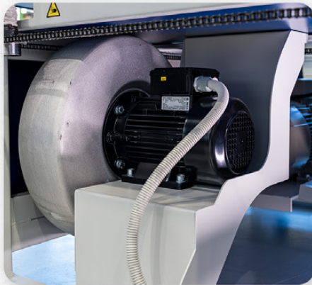
In der Maschine eingebautes Vakuumgebläse
